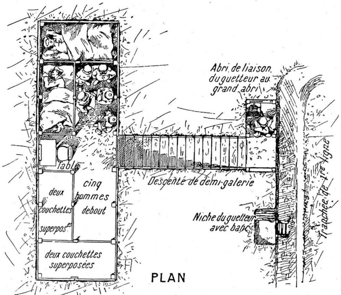
Type d'abri allemand en première ligne, avec accès par une demi-galerie en escalier.
