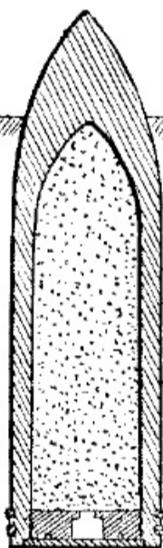
OBUS du Mortier de 305
