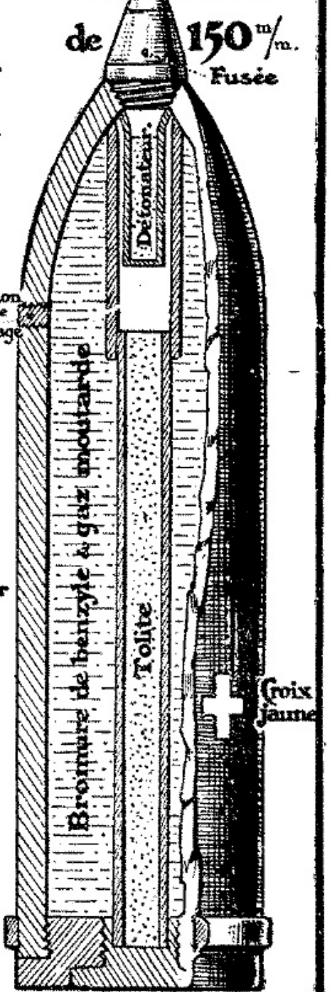
Obus Lacrymogène et vésicant de 150 m .
