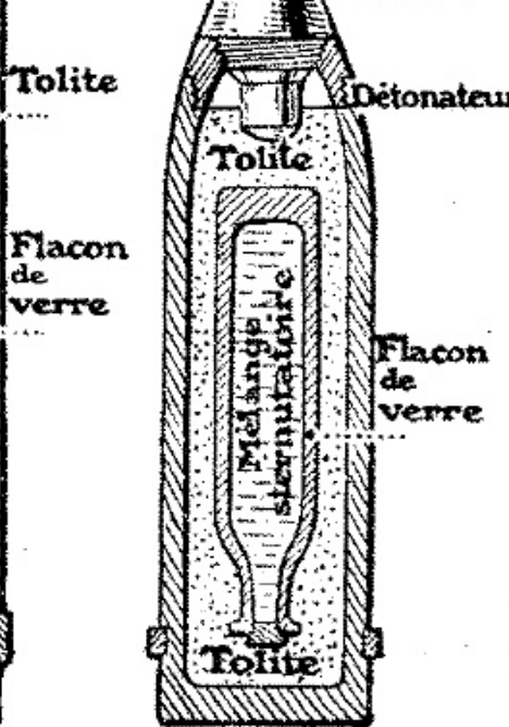
Obus de campagne de 77 m à croix bleue
